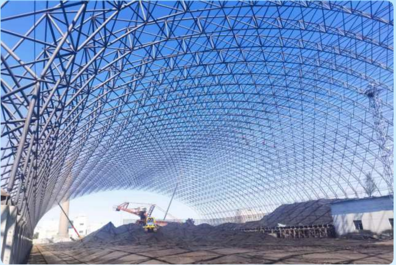
■ 储煤场网架项目 / Coal Storage Yard Grid Project
